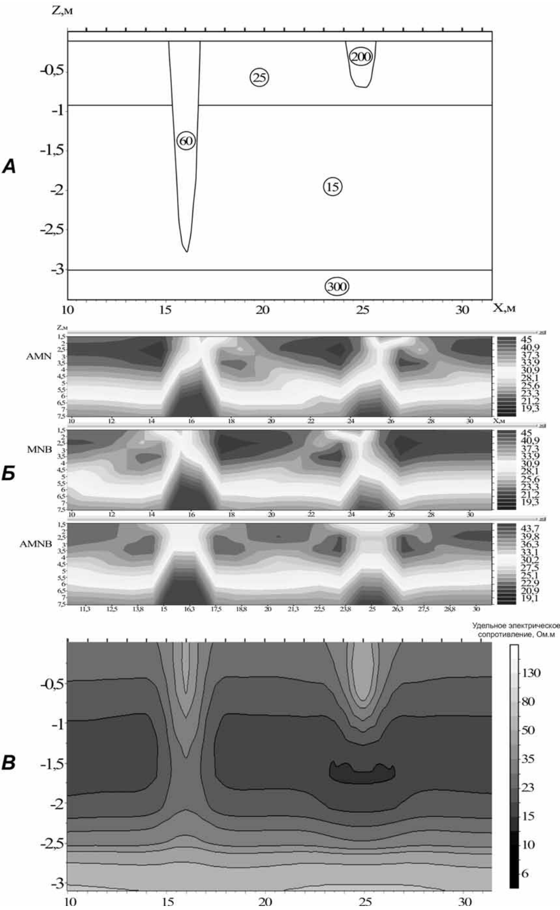
Рис. 3. Двумерное моделирование проявления на разрезах инверсии аномалий различной глубины для методики с шагом 1 м: А — геоэлектрическая модель среды (указаны значения УЭС); Б — псевдоразрезы кажущегося сопротивления для трехэлектродных установок Амн и mnВ и четырехэлектродной установки АмнВ; В — геоэлектрический разрез по результатам инверсии
