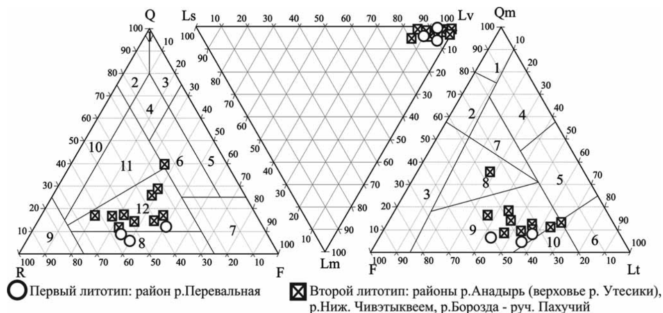
Рис. 4. Диаграмма минерального состава песчаников В.Д. Шутова [Шутов, 1972] (А): Q — кварц, F — полевые шпаты, R — литокласты: 1 — мономинеральные кварцевые, 2 — кремнекласитикварцевые, 3 — полевошпатово-кварцевые, 4 — мезомикто-кварцевые, 5 — собственно аркозы, 6 — граувакковые аркозы, 7 — поле пород не терригенного происхождения, 8 — полевошпатовые граувакки, 9 — собственно граувакки, 10 — кварцевые граувакки, 11 — полевошпатово-кварцевые граувакки, 12 — кварцево-полевошпатовые граувакки; Диаграмма эволюции состава обломков пород (Б): Lm — обломки метаморфических пород (кварциты), Ls — обломки пород осадочного происхождения, Lv — обломки вулканических пород; а также треугольная диаграмма (В) Qm—F—Lt (Qm — кварц монокристаллический, F — полевой шпат, Lt — все обломки пород, включая поликристаллический кварц Qp), по [Dickinson, Suczek, 1979]: 1 — породы древних платформ, преимущественно кварцевые; 2 — окраинных морей, полевошпатово-кварцевые; 3 — породы выступов кристаллического фундамента, полевошпатовые; 4 — кварцевые переработанные, кварцевые литические; 5 — переходные переработанные, кварцевые литические; 6 — литические переработанные, литические; 7 — смешанные; 8 — расчлененных островных дуг, полевошпатово-литические; 9 — переходных островных дуг, литически полевошпатовые; 10 — нерасчлененных (активных) островных дуг, литические.
