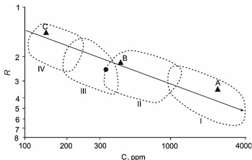
Рис. 9. Диаграмма R–Cr для определения типа материнских пород с фигуративной точкой составов изученных бокситовых образований, по [Özlü, 1983]. А, В и С — составы латеритов по амфиболитам, базальтам и гранитам соответственно. Типы материнских пород: ультраосновные (I), основные (II), среднего состава или глинистые (III), кислые (IV)
