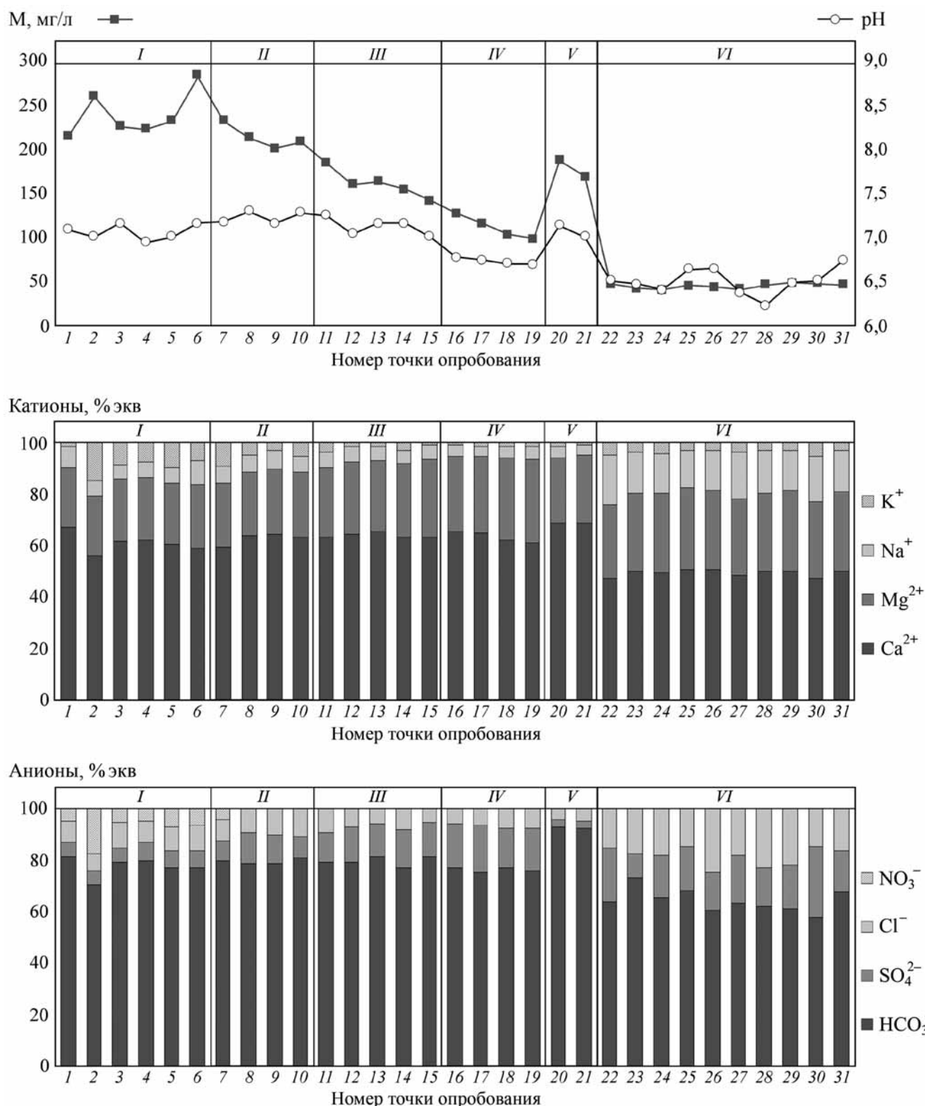
Рис. 2. Минерализация, pH и ионный состав поверхностных вод: I — канал имени Москвы, II — Угличское вдхр, III — Рыбинское вдхр, IV — Шекснинское вдхр, V — вдхр Волго-Балтийского канала (Вытегорское и Белоусовское), VI — Онежское озеро
