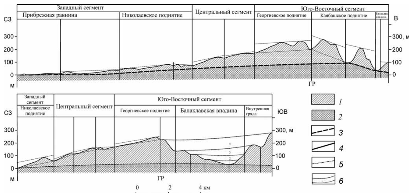
Рис.7. Геоморфологические профили через Гераклеийский полуостров: А — по линии 1–1'. Б — по линии 2–2'. 1 — массив, затронутый эрозийным расчленением; 2 — массив, не затронутый процессами эрозии; 3 — сопоставительная линия, объединяющая глубину эрозийного расчленения крупными реками; 4 — границы блоков, установленные по геоморфологическим данным; 5 — региональные циклы эрозийного расчленения; 6 — сопоставительные линии реконструкции горного сооружения; 7 — зона Георгиевского разлома
