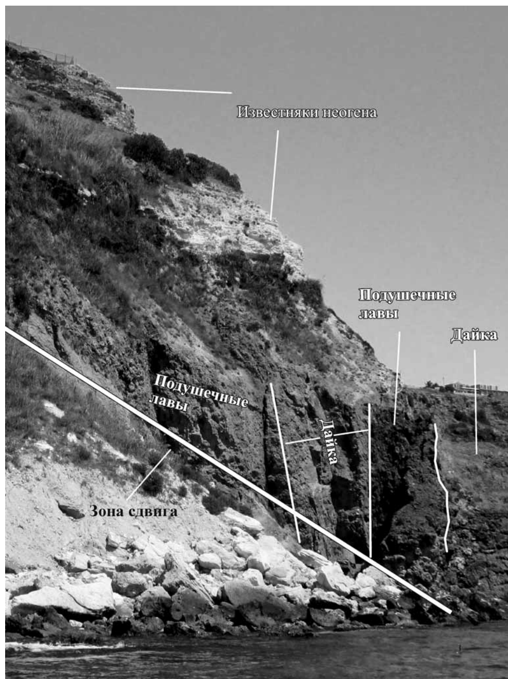
Рис. 2. Активизированная зона сдвига северо-западного простираения в районе мыса Броневой (точка 1 на рис. 1)
